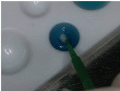
Slika 4. Ortofosforna kiselina.
