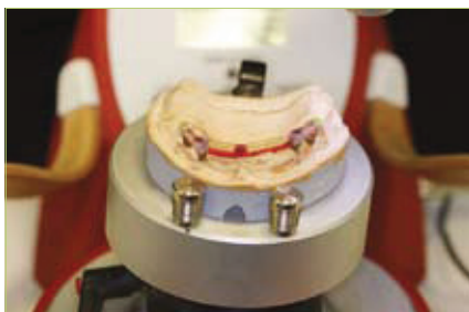
Slika 3. Radni model postavljen u ležištu paralelometra
