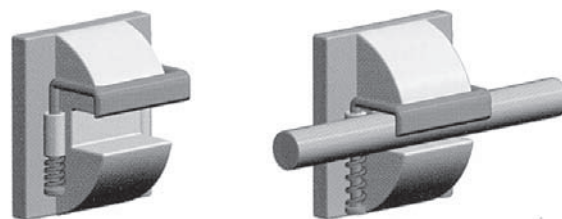
Slika 4. Boyd bravica
