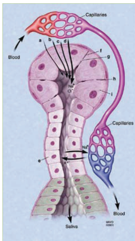
Slika 3. Lučenje sline. Primarna sekrecija zbiva se u acinusima, a aktivni transport iona u izvodnim kanalčićima. Mehanizmi kojima sastojci plazme dospijevaju u slinu:
