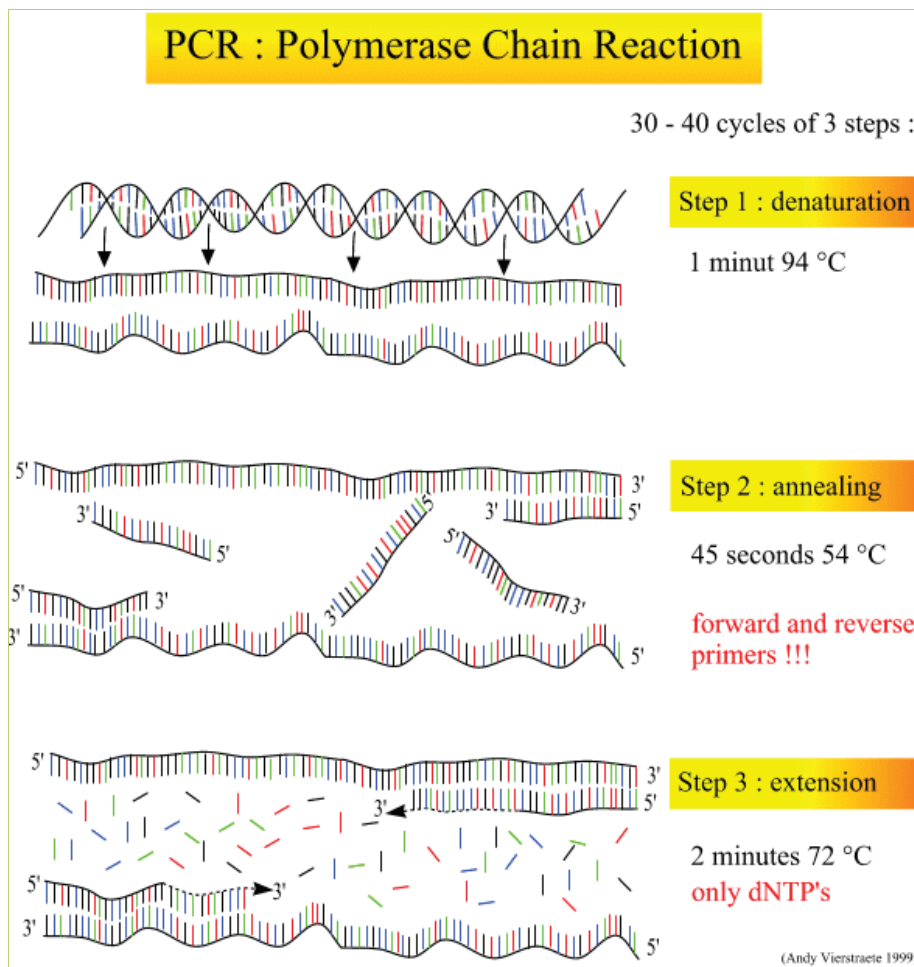
Slika 2. Izvođenje PCR
